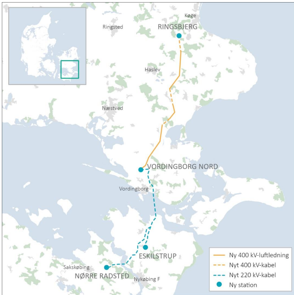
Figur 1: Skitse over Energinets planlagte projekt, Nyt elnet til Sydsjælland, Lolland og Falster.
