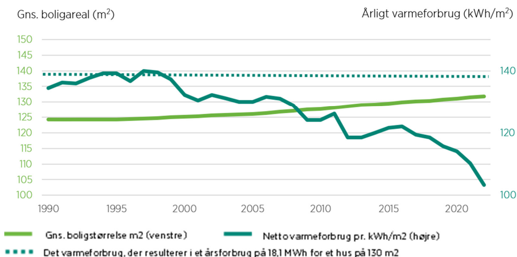
Figur 1 Estimeret historisk udvikling i gns. boligstørrelse for fjernvarmeopvarmede huse og danske husholdningers gns. årlige varmemeforbrug pr. m 2
