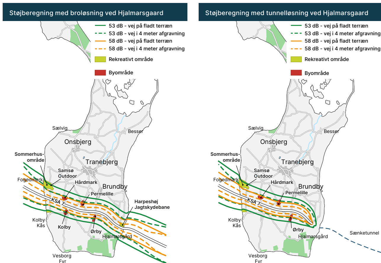
Figur 4.22 Beregning af (potentiell) støjpåvirkning på Samsø ved løsning KSA 7
