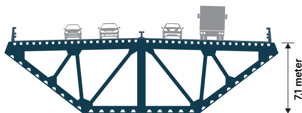
Figur 4.7 Tværsnit af bro
