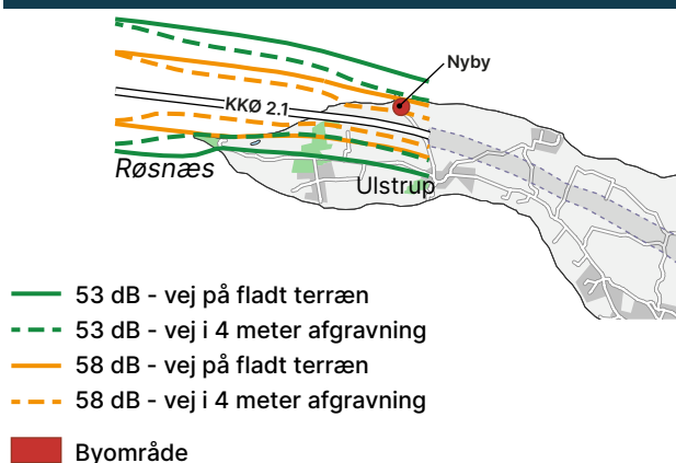
Figur 4.9 Beregning af (potentiell) støjpåvirkning på Røsnæs af broløsning i korridor KKØ 2.1
