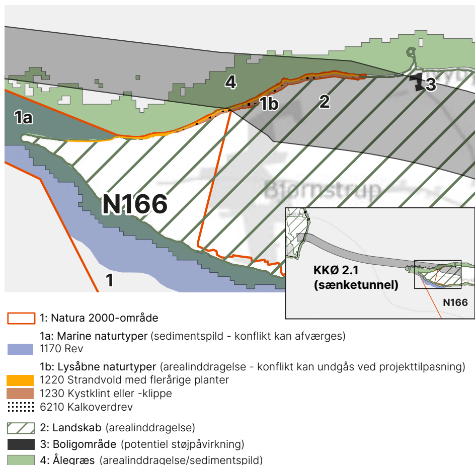
Figur 4.12 Identificerede miljøforhold ved løsning KKØ 2.1 (Sænkettunnelløsning)
