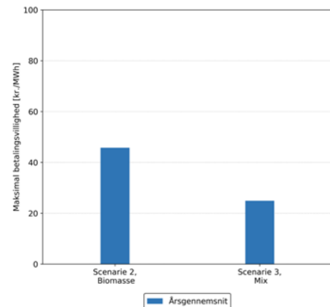
Figur C3: Maksimal betalingsvillighed for 35°C overskudsvarme på årsbasis. Betalingsvilligheden inkluderer investering i en elvarmepumpe til at hæve temperaturen på PtX-varmen til fremløbstemperaturen på fjernvarmeværket.
