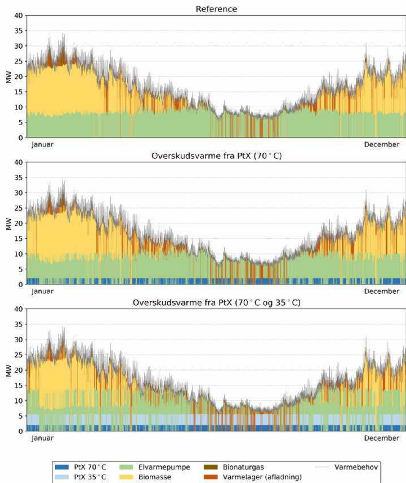
Figur 5: Sammensætning af varmeproduktionen hen over året for scenarie 3, hvor varmen primært produceres på en biomassekedel og en eldrevet varmepumpe på udeluft. Øverst ses fjernvarmesystemets driftsprofil hen over et år uden overskudsvarme fra PtX. I midten udnyttes overskudsvarmen ved 70 °C, hvilket fortrænger produktion på biomassekedlen og elvarmepumpen. Nederst udnyttes overskudsvarmen ved både 70 °C og 35 °C, og den udgør knap 20 % af den årlige varmeproduktion.
