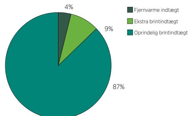
Figur 9. Følsomhedsanalyse: Fordeling i estimerede indtægter for hhv. brint og fjernvarme ved en værdi af varmen på hhv. 110 kr./MWh om sommeren og 180 kr./MWh om vinteren for 70 °C. Værdien af varmen ved 35 °C aftages til 0 kr./MWh.
