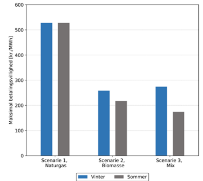
Figur C2: Den maksimale betalingsvillighed for udnyttelse af 70 °C overskudsvarme fra PtX for de tre fjernvarmesystemer. Scenarie 2 og 3 har forskellig betalingsvillighed sommer og vinter, da der fortrænges dyrere varmeproduktion om vinteren end om sommeren. Scenarie 1 har en høj, beregnet maksimale betalingsvillighed, som ikke svarer til den pris, som PtX-anlægget kan sælge varmen til. Det indikerer derimod, at fjernvarmesystemet står over for en omstilling, hvor varmeprisen kan reduceres gennem investeringer i billigere varmeproduktion. En af disse muligheder er overskudsvarme fra PtX.
