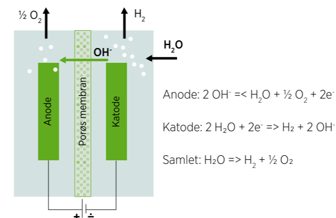
Figur A1. Alkalisk elektrolyse – princip og reaktioner
