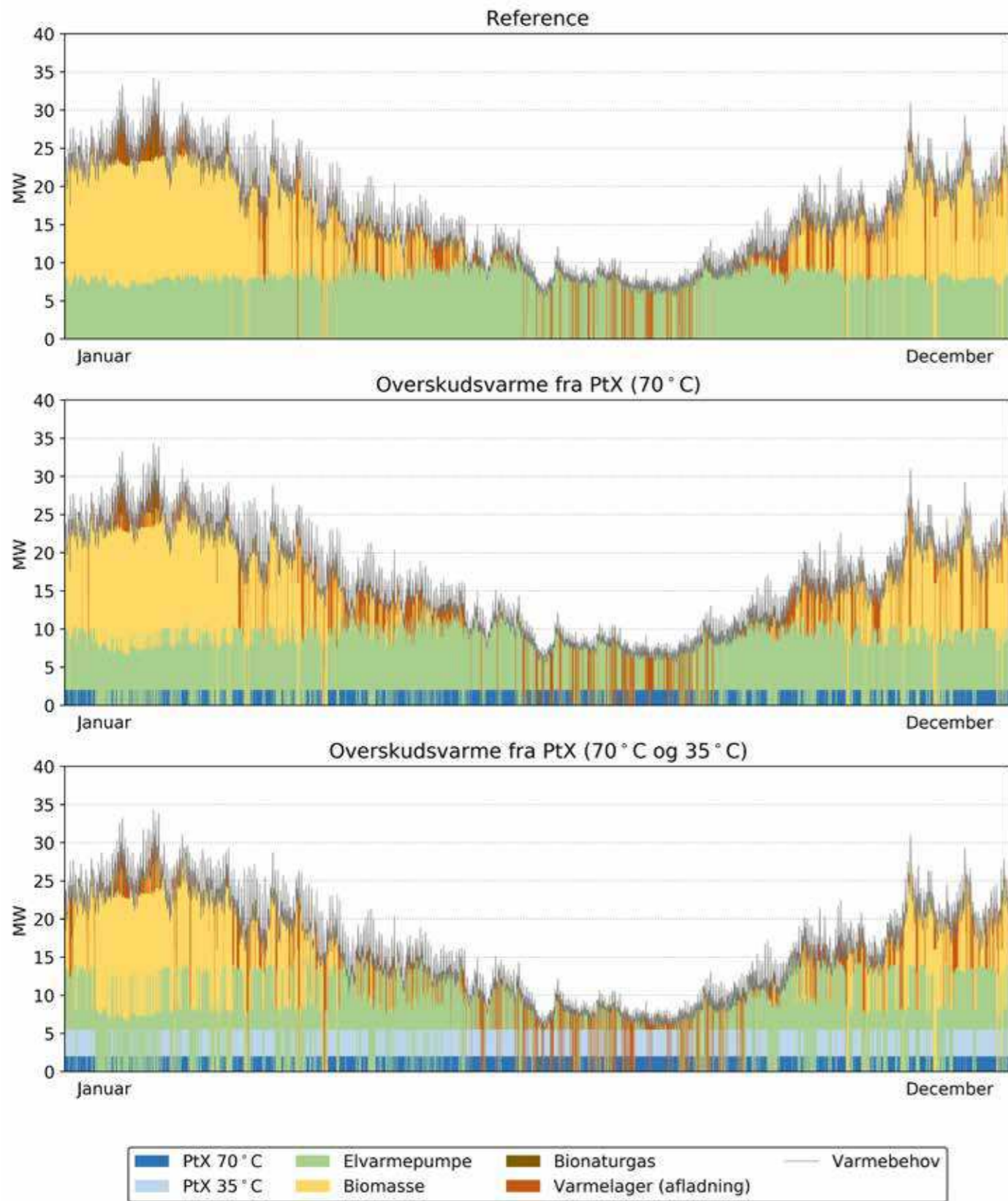
Figur C1: Sammensætning af varmeproduktionen hen over året for scenarie 3, hvor varmen primært produceres på en biomassekedel og en eldrevet varmepumpe på udeluft. Øverst ses fjernvarmesystemets driftsprofil hen over et år uden overskudsvarme fra PtX. I midten udnyttes overskudsvar-
