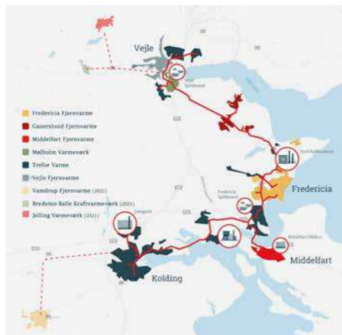
Figur 19. Varmetransmission i Trekantområdet forbinder varmeproduktion og lokale fjernvarmeområder via TVIS' fjernvarmenet (røde linjer). Kilde: TVIS.net
