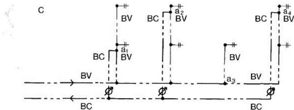
Figur 6 Eksempel på en typisk rørføring til varmt brugsvand med synlig rørføring i kælder, og stigstreng ført i rørskakte til hver enkelt lejlighed.
