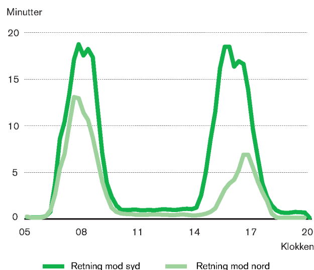
Figur 2.1. Forsinkelse i minutter pr. køretøj på E47/Motorring 3 Lundtofte-Gl. Køge Landevej på tirsdage, onsdage og torsdage, efterår 2016
