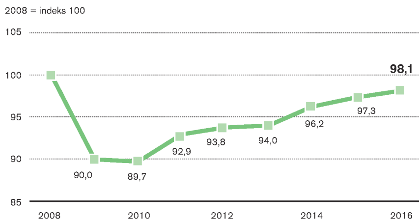
Figur 3.2. Vejdirektoratets lastbilindeks, 2008-2016
