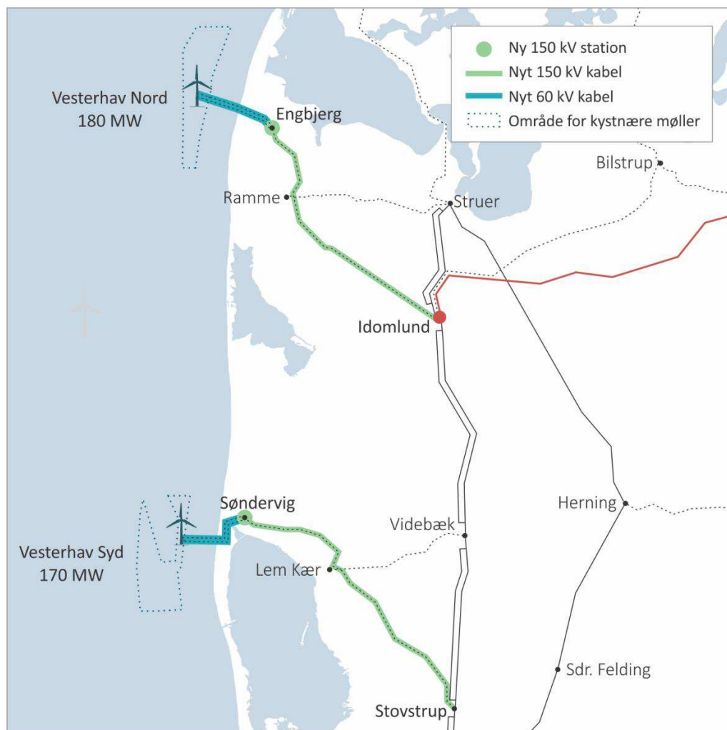
Figur 1. Placeringen i Vestjylland af nettilslutningen af de kystnære havvindmølleparker Vesterhav Nord og Vesterhav Syd.
