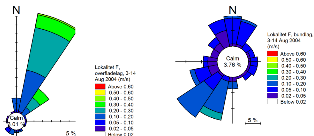
Figur 4-2 Strømhastigheder i overfladelaget (tv) og bundlaget (th) ved Standardhavbrug F i en periode med vind fra øst (3.-14. august). Baseret på MIKE3FM hydrodynamisk modellering.
