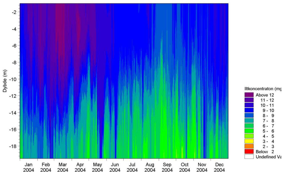
Figur 4-15 Isopleth-diagram af iltkoncentration ved Standardhavbrug F i 2004. Baseret på MIKE 3FM ECO basismodellering.
