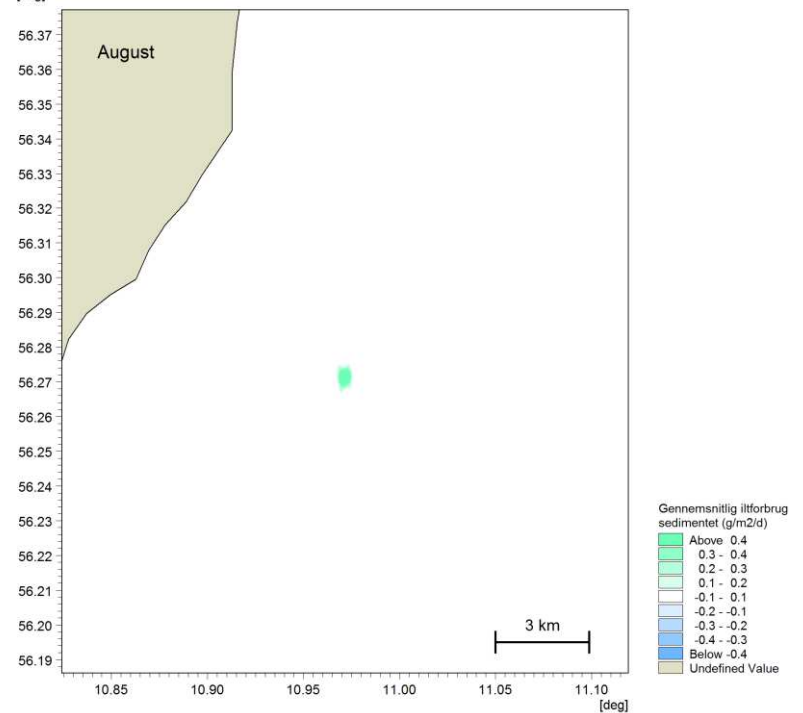
Figur 5-12 Beregnet gennemsnitlig ændring i sedimentets daglige iltforbrug i produktionssæsonen (øverst), og i august, hvor ændringen er størst (nederst). Figurer for produktionssæsonen og alle måneder er vist i Bilag I.
