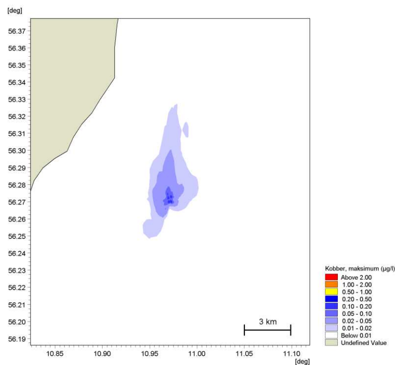
Figur 6-2 Maksimale overkoncentrationer i overfladen (0-5 m) af kobber ( \mu\text{g Cu/L} ) for perioden april-august. Overkoncentrationerne forekommer omkring Standardhavbrug F. Bemærk at figuren ikke repræsenterer koncentrationen på et bestemt tidspunkt, men den maksimale koncentration beregnet for hver gridcelle i løbet af april-august.
