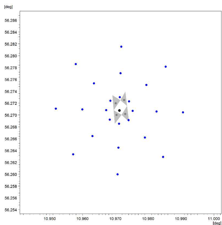
Figur 5-2 Positioner (•) for modeludtræk af data til beregning af næringskoncentrationer 50, 500 og 1000 m fra Standardhavbrug F. De fire skraverede trekanter repræsenterer området hvor burene og næringsstofkilder er lokaliseret.
