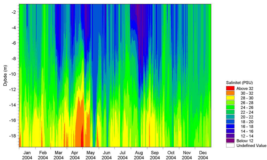
Figur 4-3 Isopleth-diagram af et års variation i salinitet ved Standardhavbrug F i 2004. Baseret på MIKE3FM hydrodynamisk basismodellering.
