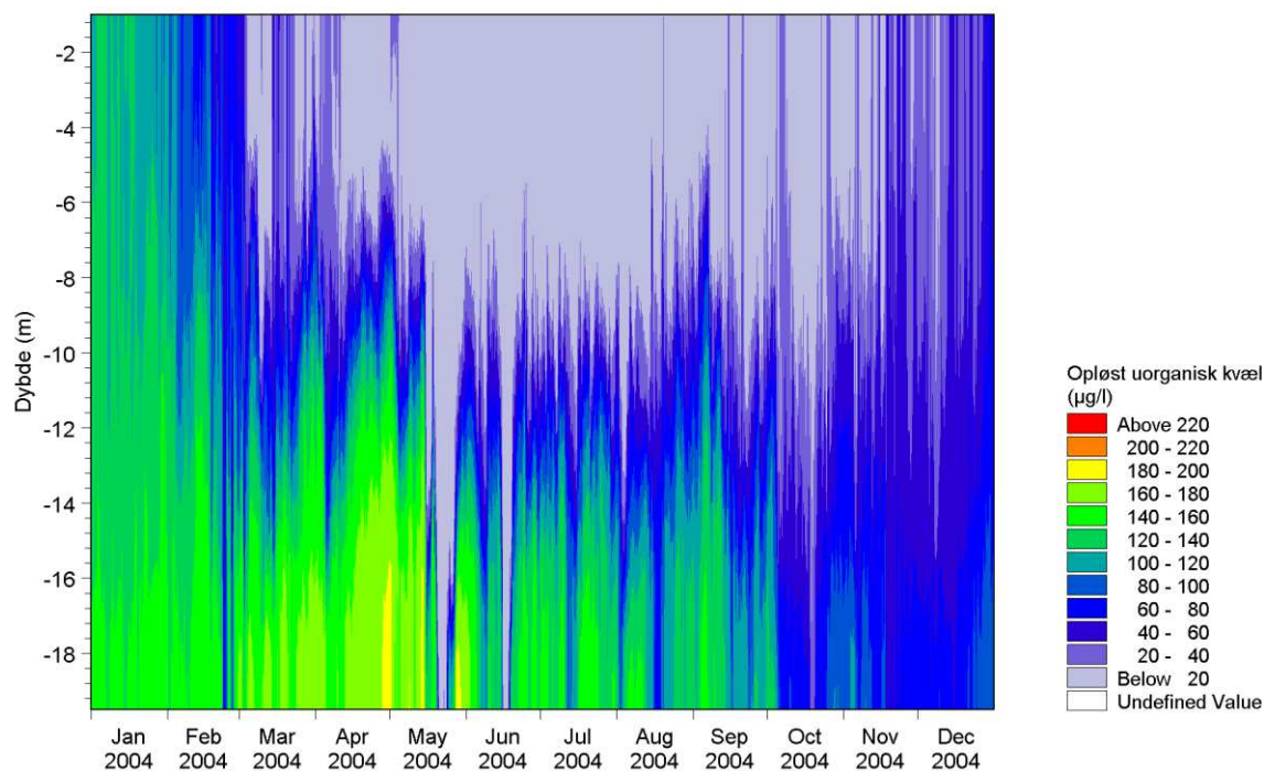
Figur 4-6 Isopleth-diagram af uorganisk kvælstof ved Standardhavbrug F i 2004. Baseret på MIKE 3FM ECO basismodellering.
