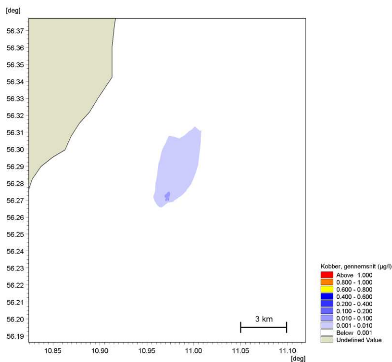
Figur 6-1 Middeloverkoncentration i overfladen (0-5 m) af kobber ( \mu\text{g Cu/L} ) i perioden april-august, hvor Standardhavbrug F anvender ny-imprægnerede net.
