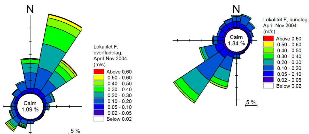
Figur 4-1 Strømroser repræsenterende retning og hastigheder i overfladelaget (tv) og i bundlaget (2 m over bunden) ved Standardhavbrug F i produktionsperioden. Baseret på MIKE3FM hydrodynamisk modellering.
