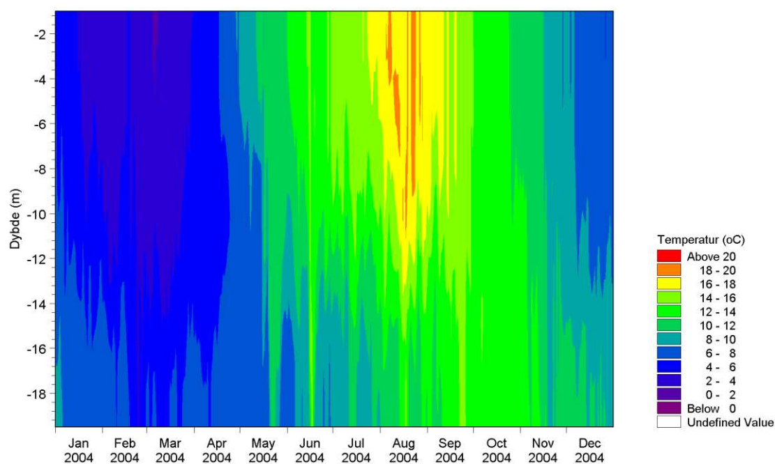
Figur 4-4 Isopleth-diagram af temperatur ved Standardhavbrug F i 2004. Baseret på MIKE3FM hydrodynamisk basismodellering.
