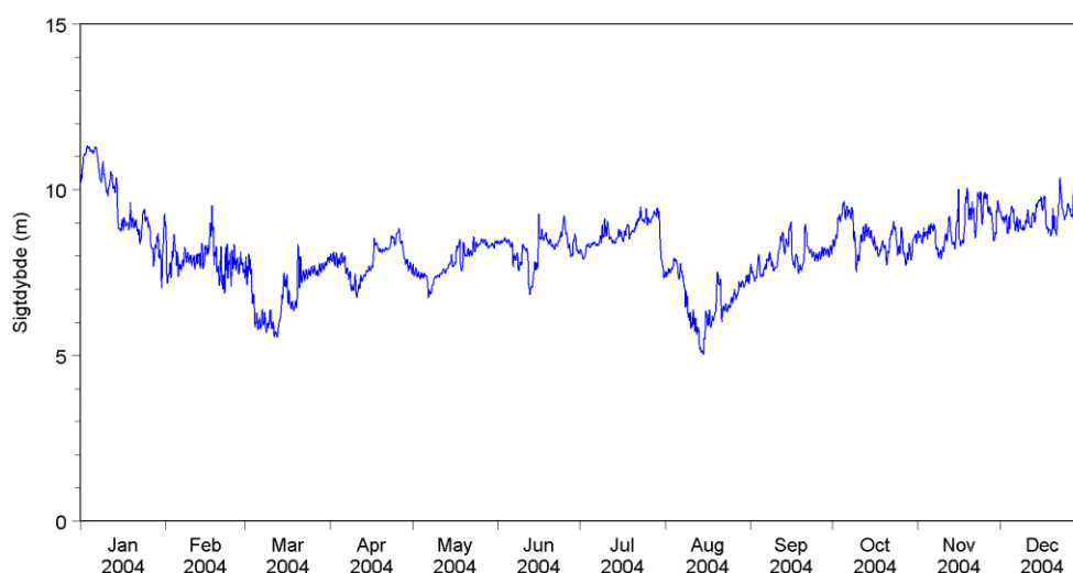
Figur 4-13 Tidsserie af sigtdybde ved Standardhavbrug F. Baseret på MIKE 3FM ECO basismodellering.
