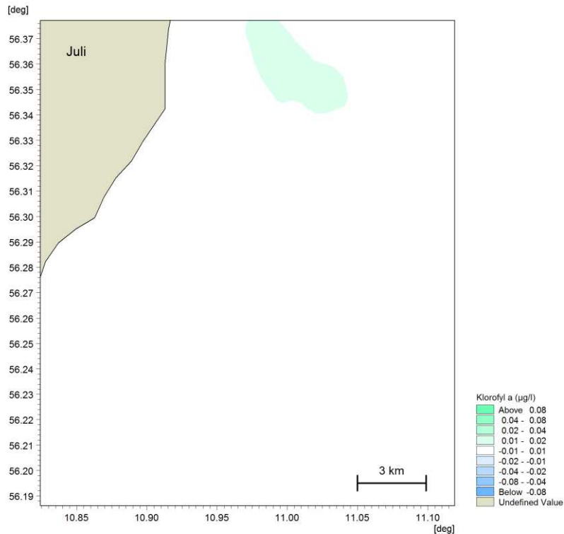
Figur 5-7 Beregnet gennemsnitlig ændring i koncentrationen af klorofyl i overfladen omkring Standardhavbrug F i produktionssæsonen (øverst) og i juli, hvor ændringen er størst (nederst). Til venstre er vist et oversigtskort og til højre et zoom på det område, hvor der beregnes ændringer i primærproduktionen. Figurer for produktionssæsonen og de enkelte måneder i denne findes i Bilag D
