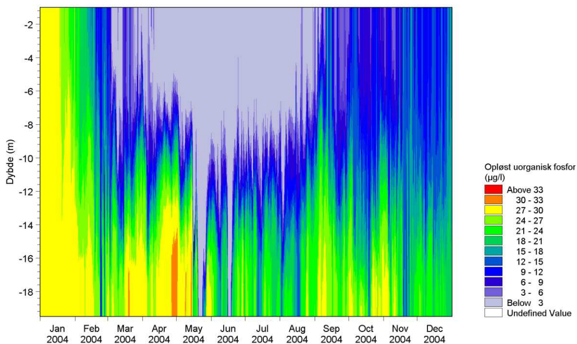
Figur 4-7 Isopleth-diagram af uorganisk fosfor ved Standardhavbrug F i 2004. Baseret på MIKE 3FM ECO basismodellering.
