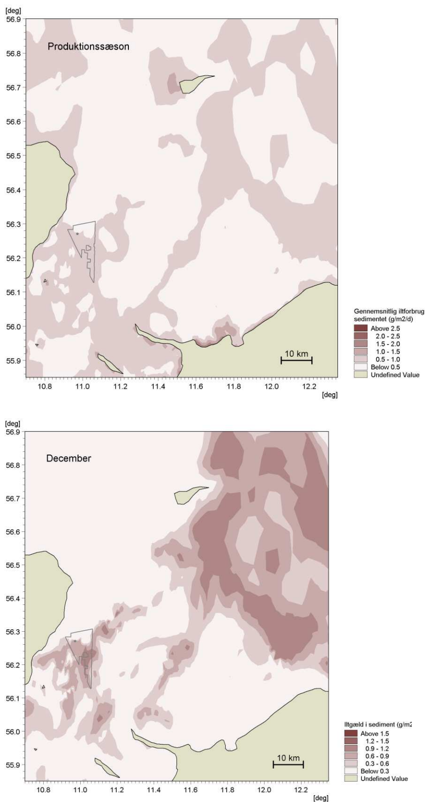
Figur 4-20 Gennemsnitlige iltforbrug i sedimentet i perioden april-december (øverst) og iltgæld i sedimentet (nederst) ultimo december. Baseret på MIKE 3FM ECO basismodellering. Lokalisering af Havbrugszone F / Standardhavbrug F er vist.
