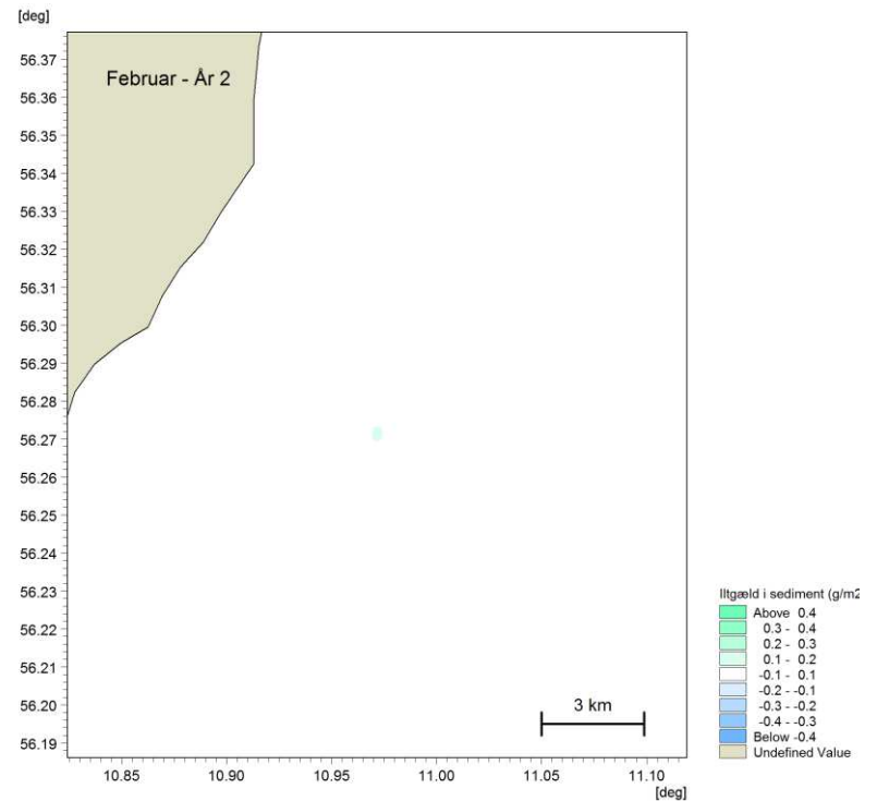
Figur 5-13 Beregnet gennemsnitlig ændring i sedimentets iltgæld ( \text{g/m}^2 ) i produktionssæsonen (øverst) og i august, hvor ændringen er størst (midt) og i februar den efterfølgende brakperiode, som er sidste måned med ændring (nederst). Figurer for produktionssæsonen og alle måneder er vist i Bilag K.
