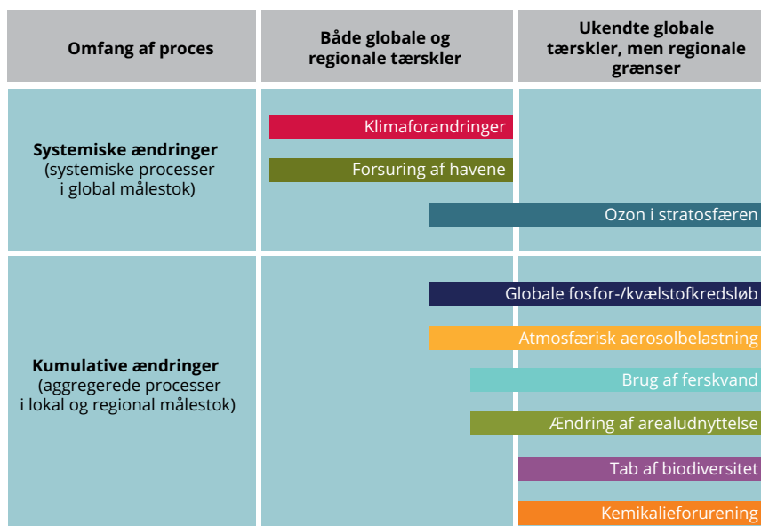
Figur 2.5 Kategorier af planetære grænser
