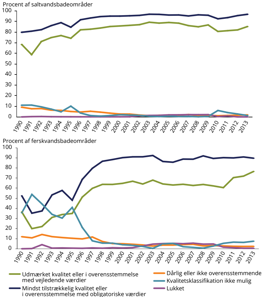
Figur 5.1 Kvaliteten af saltvands- (øverst) og ferskvandsbadeområder (nederst) i Europa, 1990-2013
