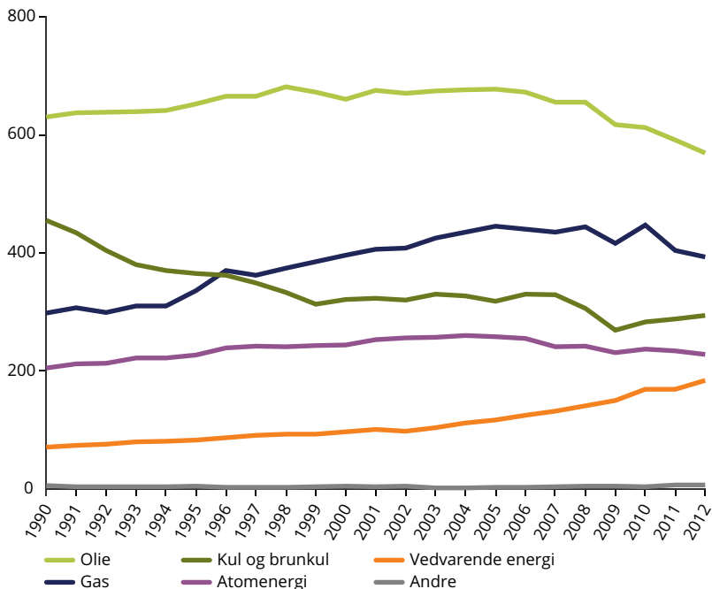
Figur 4.5 Bruttoenergiforbrug efter brændstof (EU-28, Island, Norge og Tyrkiet), 1990-2012
