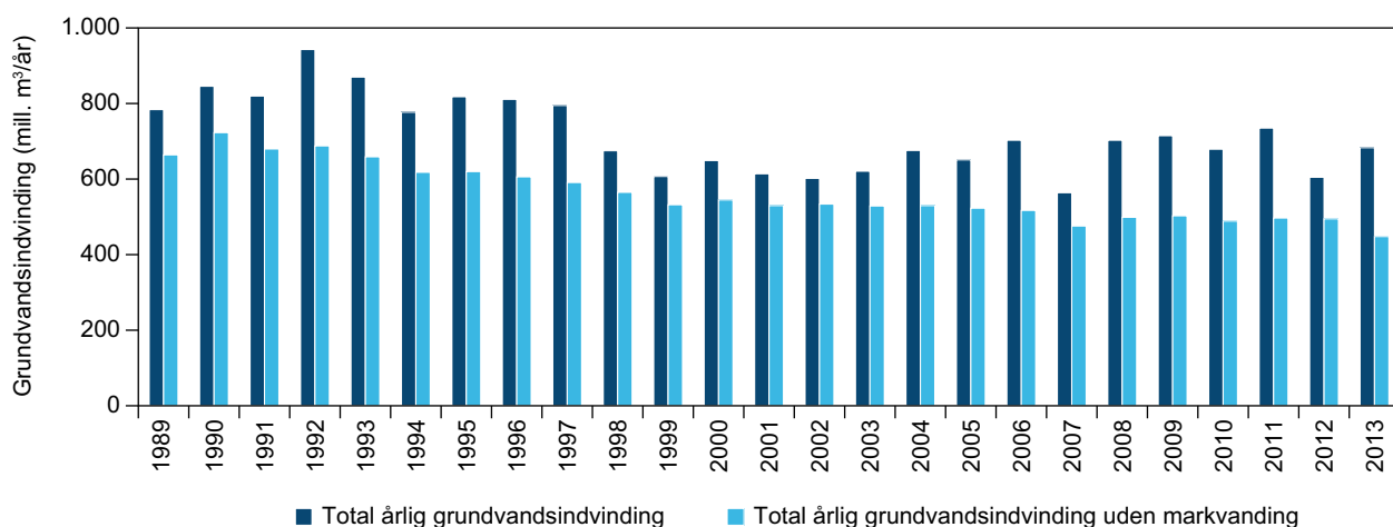
Figur 6.2. Den samlede grundvandsindvinding med og uden markvanding i Danmark i 1989-2013. Data fra 2013 er foreløbige på grund af ufuldstændig indberetning (Thorling et al. 2015).
