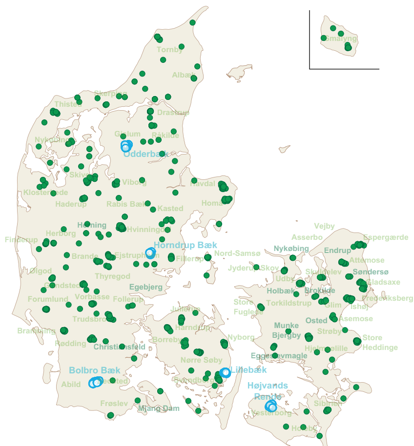
Figur 6.1. Stationsnettet for vandanalyser til grundvandsovervågningen i 2013. (Thorling et al. 2015).
