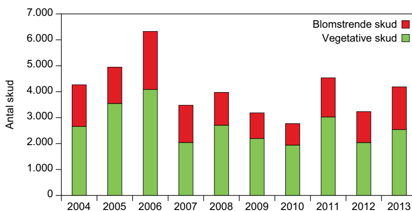
Figur 10.4. Den samlede bestandsudviklingen af mygblomst 2004-2013. Kaldred-bestand blev ikke optalt i 2007, mens der fra 2008 kun blev optalt et repræsentativt udsnit af bestanden (Søgaard et al. 2015).
