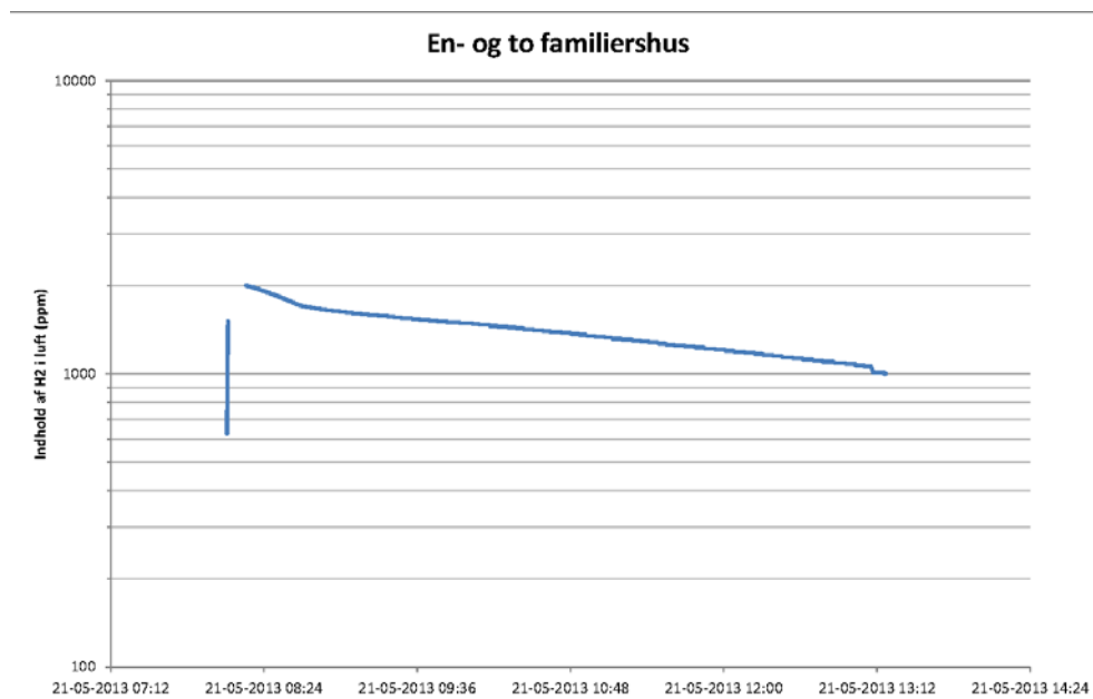
Figur 6. Målte henfald af brint efter udspredning og homogenisering i rum A. Luftskiftet beregnes som udfra kurvens hældning.
