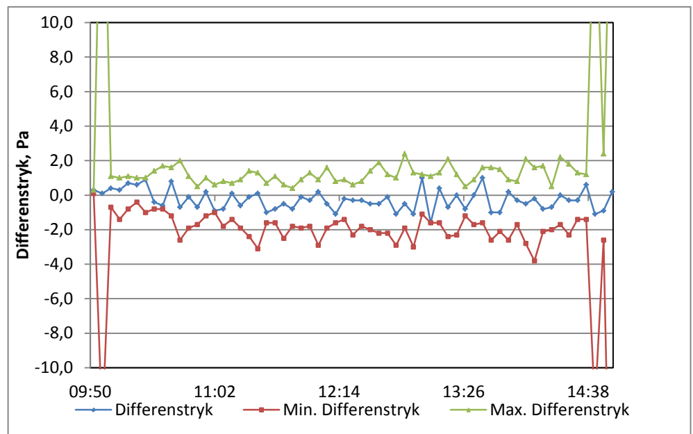
Figur 10. Trykdifferensmålinger over en måleperiode fra 9.48-14.48. Målt mellem indeluft og hulmur. Som det fremgår, er der svingende trykdifferens i bygningen i måleperioden, hvilket betyder at der er perioder med overtryk og perioder med undertryk i bygningen. Negativ trykdifferens betyder, at der er undertryk i boligen. Grøn kurve er den højeste målte positive trykdifferens i perioden mellem to dataregistreringer. Rød kurve er den højeste målte negative trykdifferens i perioden mellem to dataregistreringer. Blå kurve er trykdifferensen, der er registreret i måleperioden.
