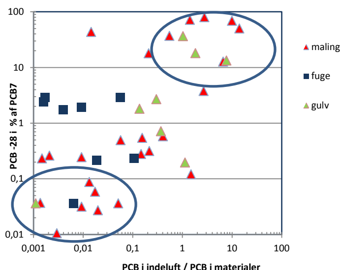
Figur 38 Andel af PCB-28 vist mod forholdet mellem PCB i indeluft ( i \text{ ng/m}^3 ) og PCB i det materiale, som antages at være hovedkilden.
