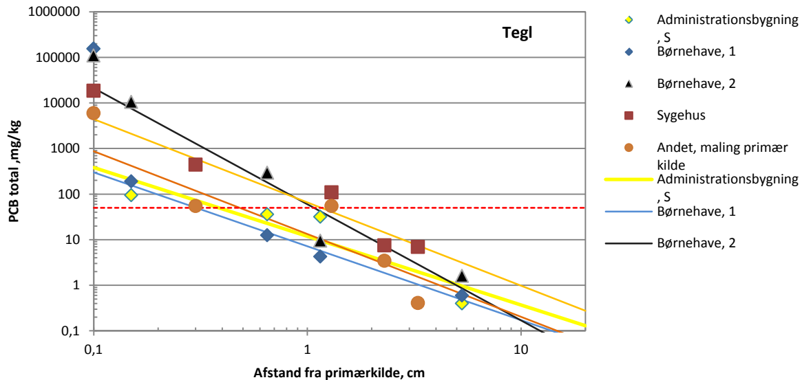
Figur 20 Målinger af PCB indtrængning i tegl i fire forskellige bygninger. Koncentrationen i primærkilden er vist som et målepunkt i 0,1 cm og indgår ikke ved beregning af regressionslinjer. Hvis andet ikke er angivet er primærkilden fugemasse. Primærkilde for "Administrationsbygning; S" er 155.000 mg/kg og gemmer sig bag markeringen for "Sygehus". Indtegnede linjer er baseret på lineær regression på de logaritmisk transformerede data.
