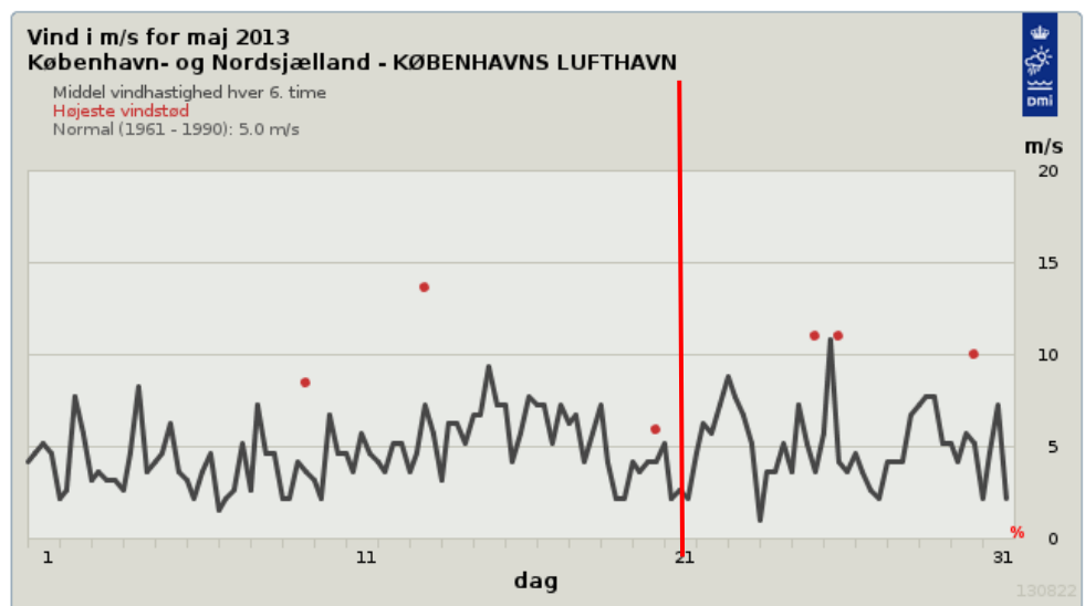
Figur 4 viser vindhastighed på prøvetagningsdagen den 21. maj 2013.
