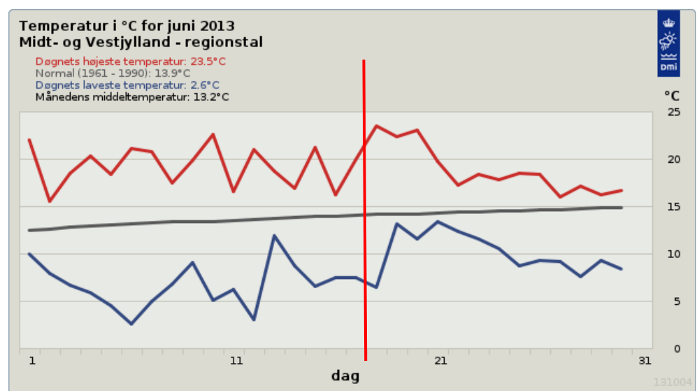
Figur 2 viser temperaturvariation på prøvetagningsdagen den 17.-18. juni 2013
