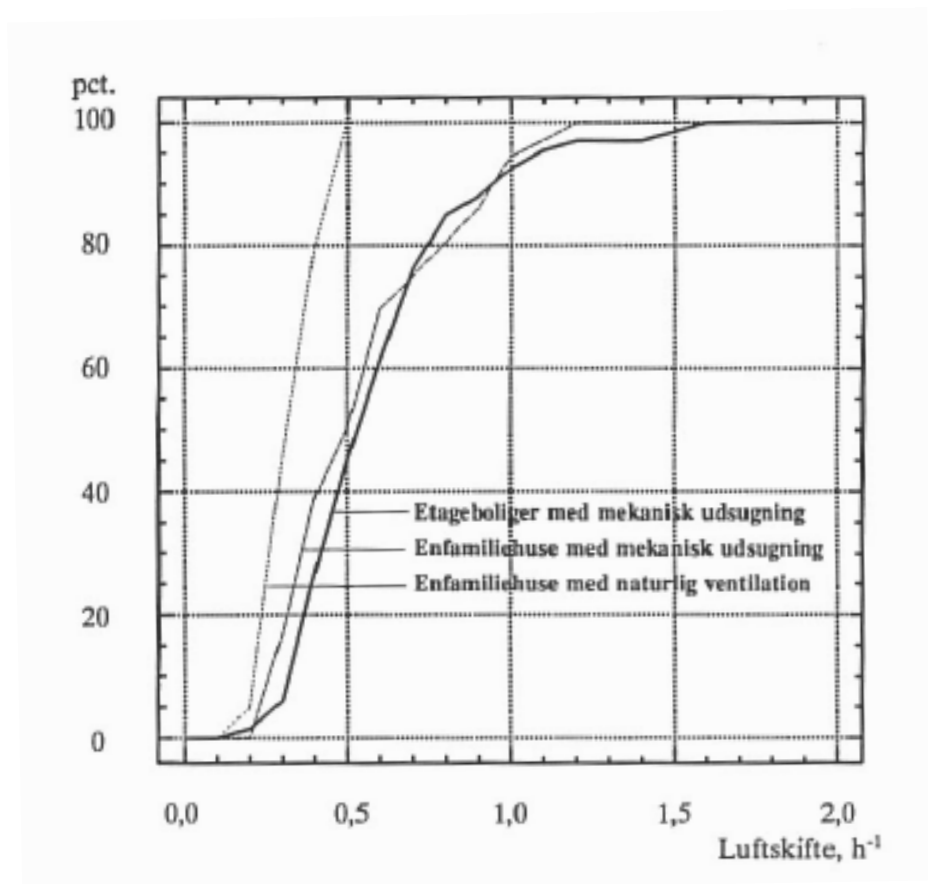
Figur B2-3. Kumuleret, relativ fordeling af udeluftskiftet i etageejendomme og enfamiliehuse.
