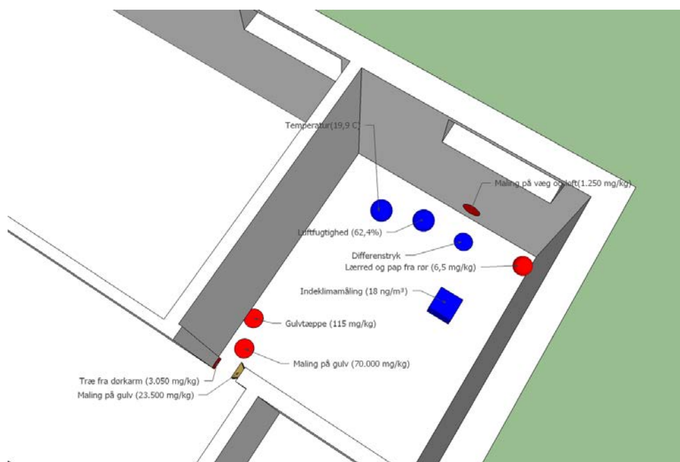
Figur 1 Målepunkter for bygningsmaterialer, indeluft, differenstrykmåling, temperatur og luft fugtighed, samt angivelse af resultat af målinger i rum A. På denne lokalitet er primær kilden maling på gulv. Maling på væg kan være en sekundær kilde eller en primær kilde. Øvrige bygningsmaterialer vurderes at være sekundære eller tertiære kilder med PCB.
