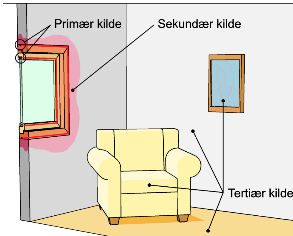
Figur 7. Principskitse for primær, sekundær og tertiære kilder i en bygning med en primærkilde af indvendige fuger. SBI-anvisning 241.
