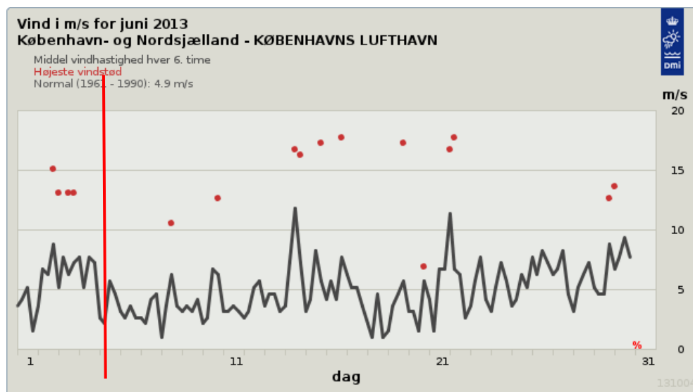
Figur 4 viser vindhastighed på prøvetagningsdagen den 5. juni 2013
