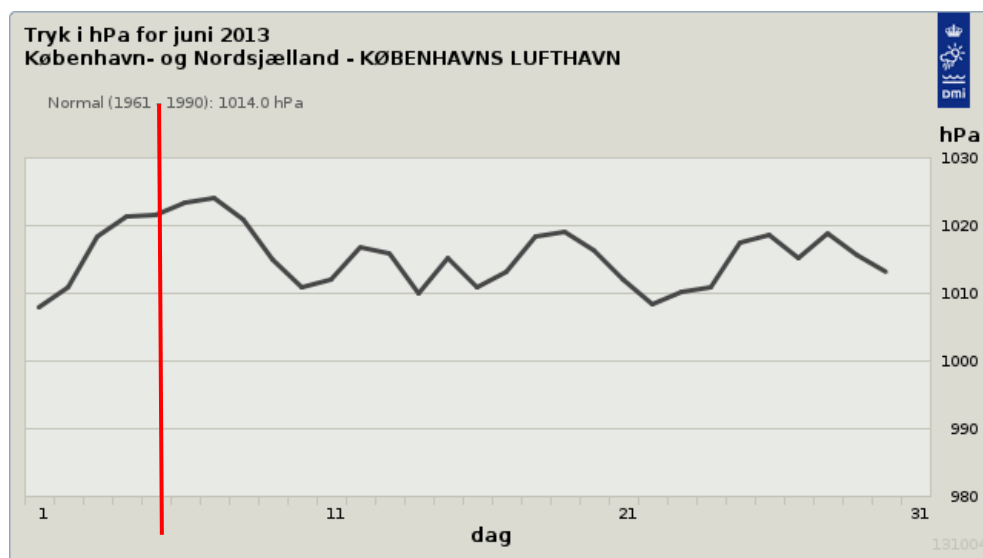
Figur 5 viser lufttrykket på prøvetagningsdagen den 5. juni 2013
