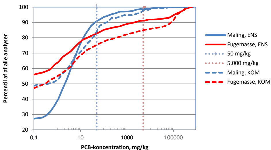
Figur 12 Kumulative fordelingsfunktioner malings- og fugeprøver.
