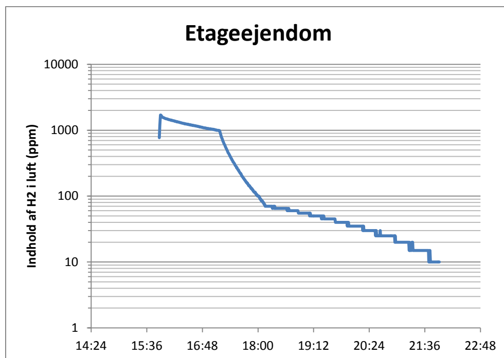
Figur 6 Målte henfald af brint efter udspredding og homogenisering i rum A. Luftskiftet beregnes ud fra kurvens hældning.
