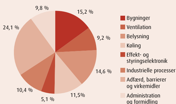
Figur 11 Elforsk-bevillinger 2002-2011
