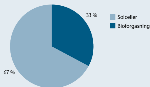
Figur 9 ForskVE-bevillinger 2011
