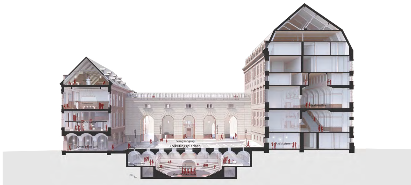
Tværsnit. Henning Larsen, JAJA Architects og Varmings Tegnestue.
