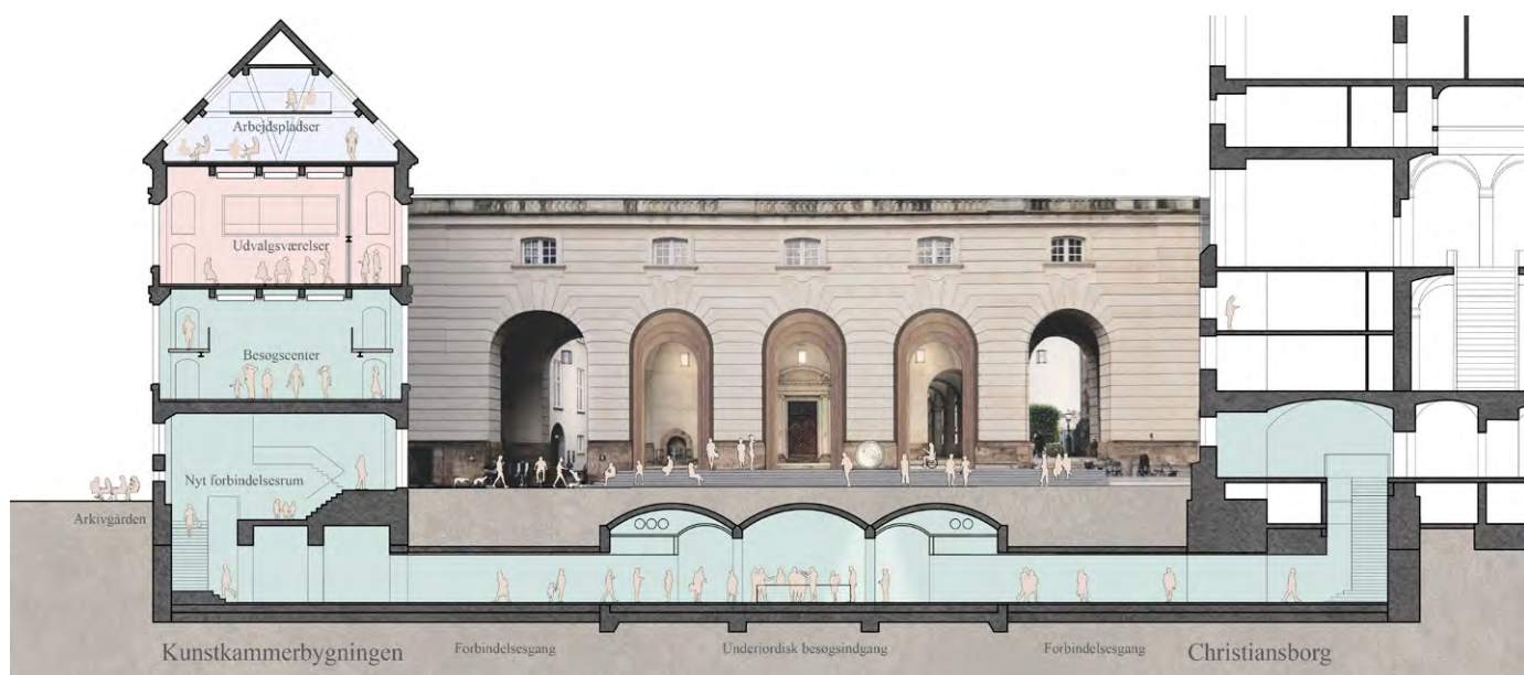
Tværsnit. Lundgaard &amp; Tranberg Arkitekter.
