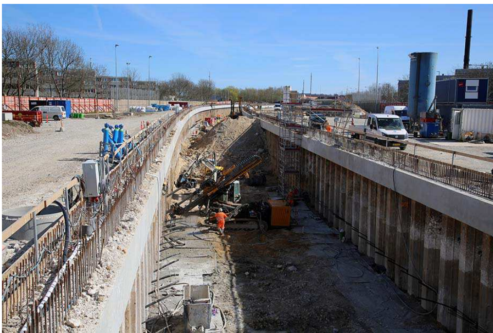
Konstruktion af trug til tunnel ved Kulbanevej i København.
