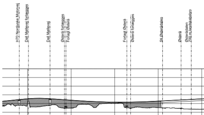
Figur 1: Længdeprofil for den 3. Limfjordsforbindelse fra E45 og frem til landskabsbroen over Østerådalen. Det mørkegrå omdeå viser, hvor motorvejen forløber på en dæmning over det eksisterende terræn
