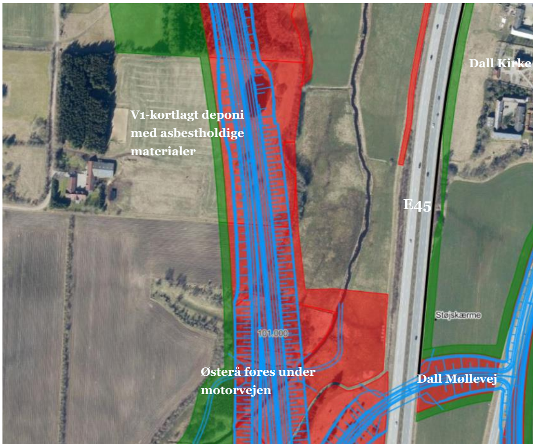
Figur 2: Den 3. Limfjordsforbindelse ved Svenstrup, hvor motorvejen forløber på dæmning over det eksisterende terræn. De røde og grønne områder er arealer, der forventes eksproprieret permanent og midlertidig i forbindelse med anlægsprojektet.
