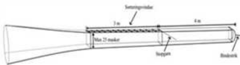
Figur 1. 4-panel fangstpose med et 180 mm kvadratmasket sorteringsvindue
