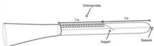
Figur 5. 2-panel fangstpose med et 180 mm kvadratmasket sorteringsvindue
