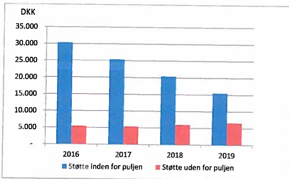
Figur 1. Støtte til husstandsmølle på 10 kW: Inden for puljen og uden puljen på 250 øre/kWh
